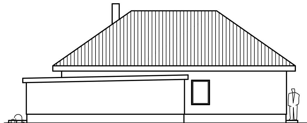
Seitenansicht Garage
