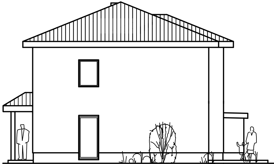
Seitenansicht
