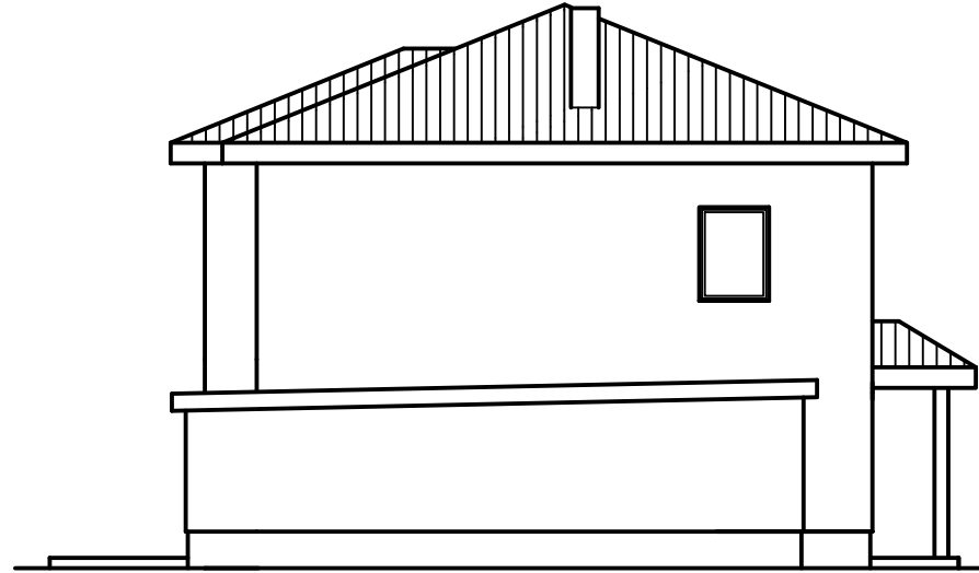
Seitenansicht-Garage
